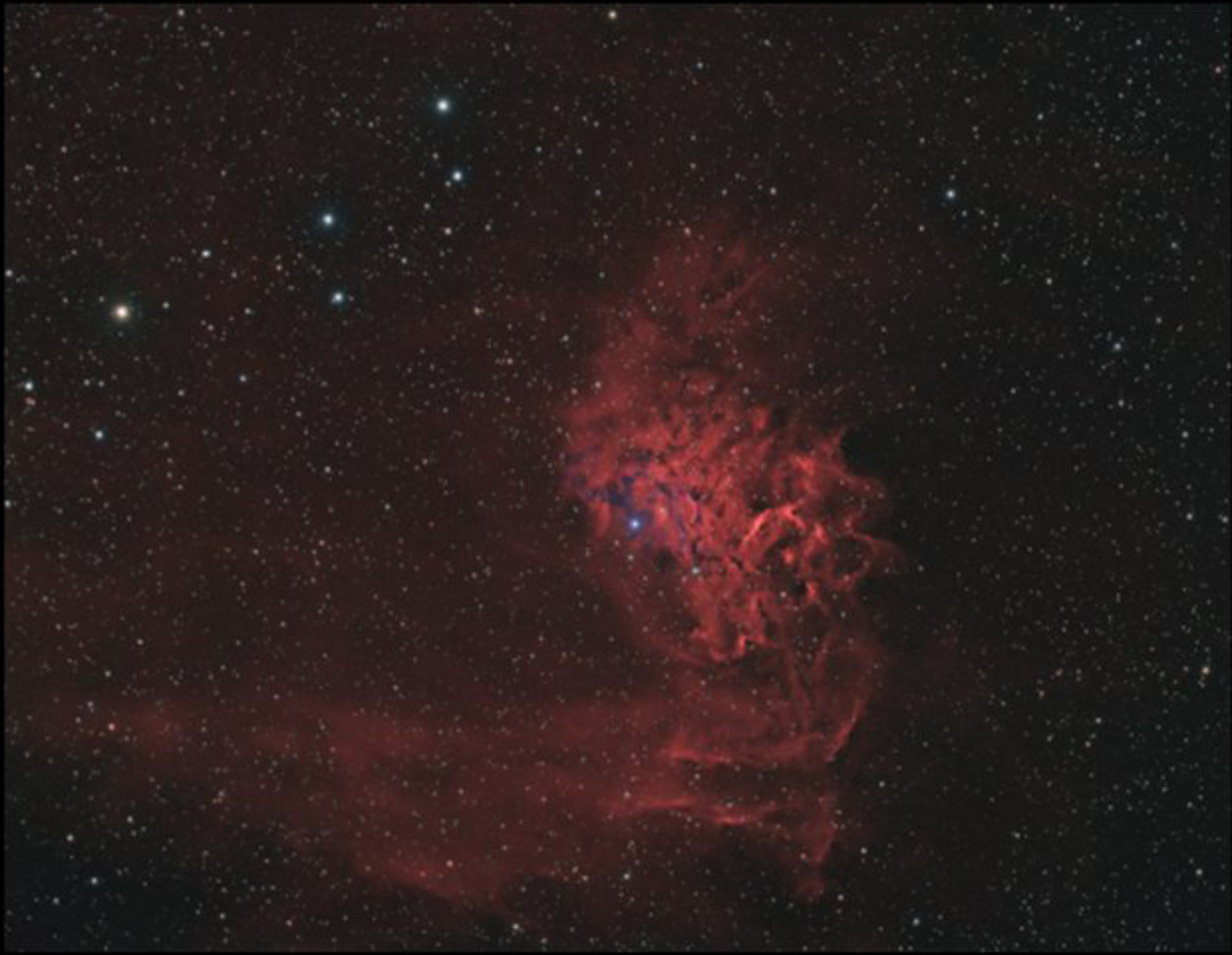
IC405 Mgławica Płonąca Gwiazda
