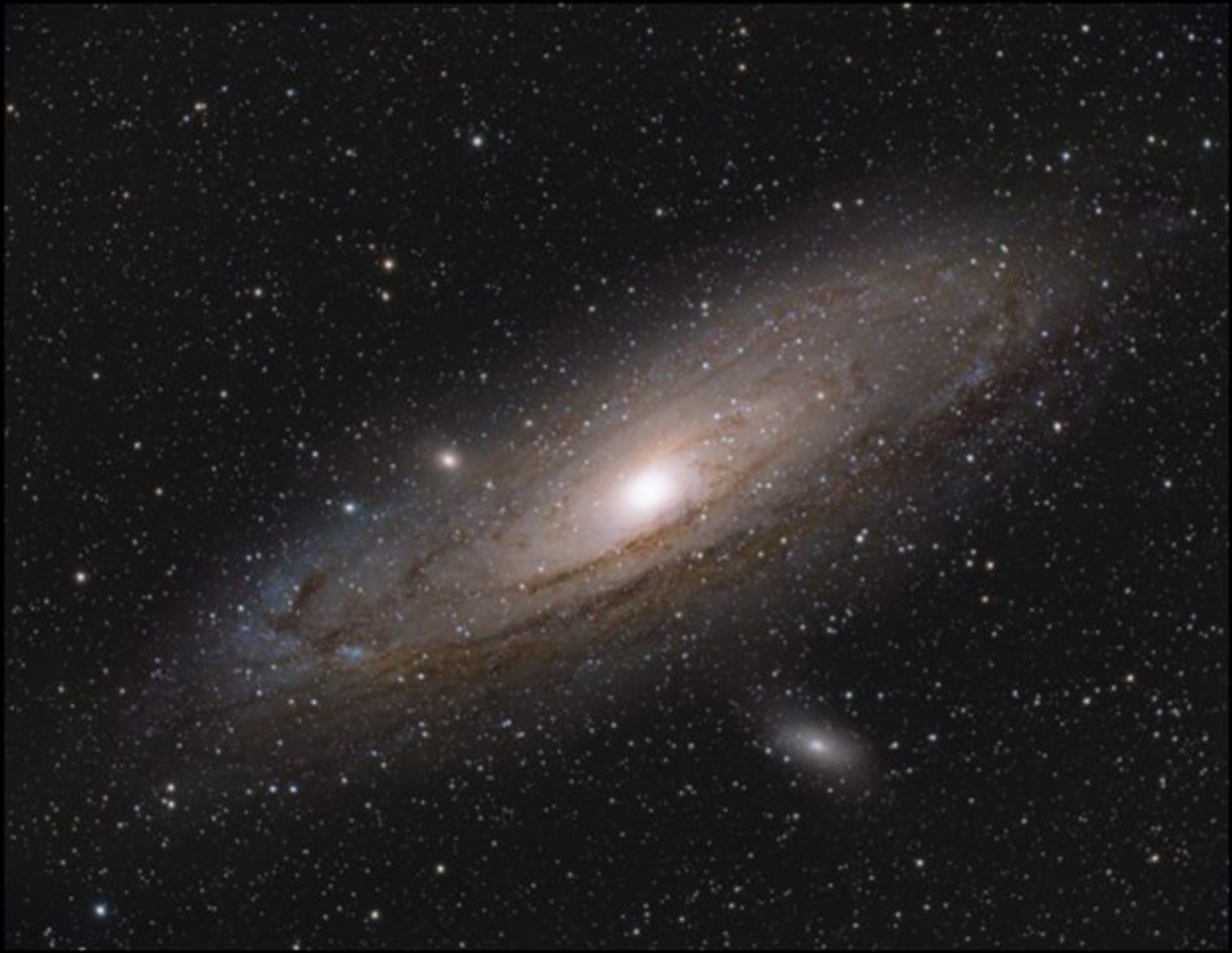
M31 Galaktyka Andromedy
